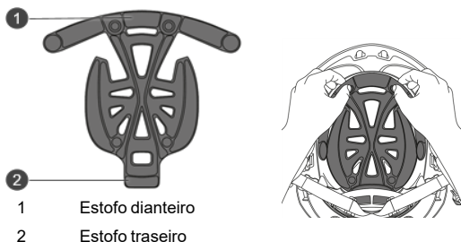
Figura 1 Estofa da suspensão
